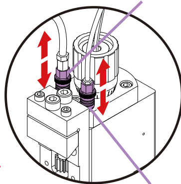
靠刀手動閥
